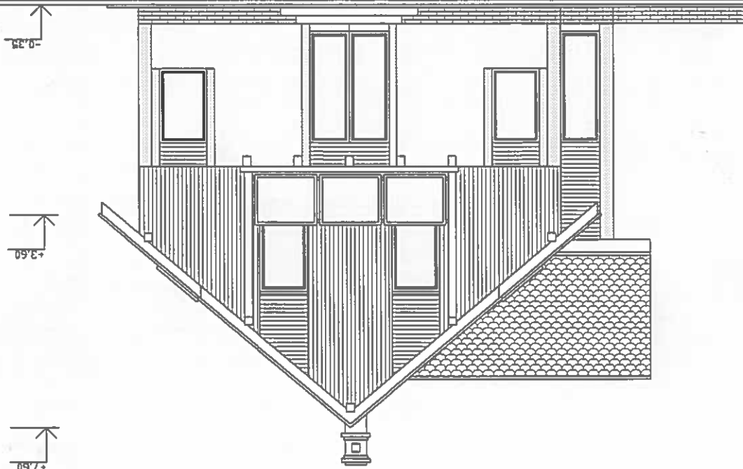
POHLAD JUHOZÁPADNÝ
