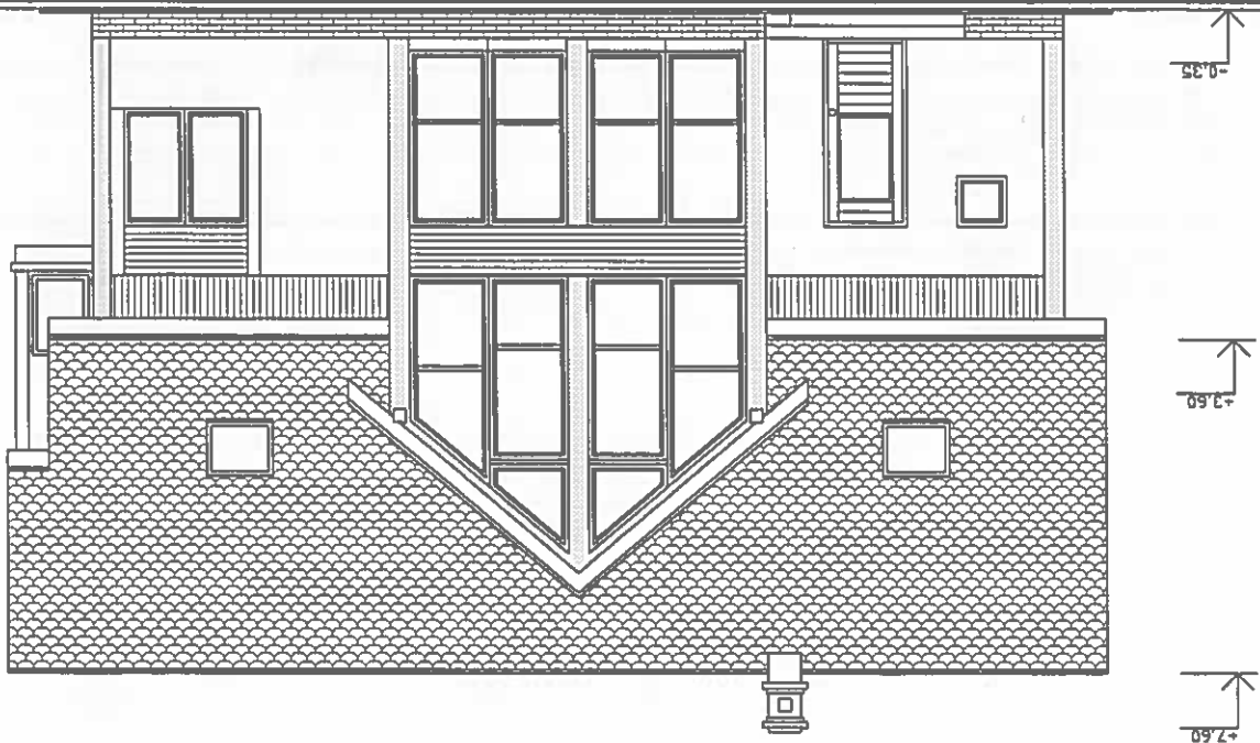
POHLAD SEVEROZÁPADNÝ
