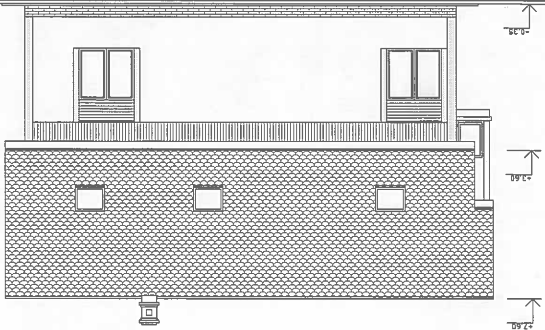
POHLAD JUHOVÝCHODNÝ
