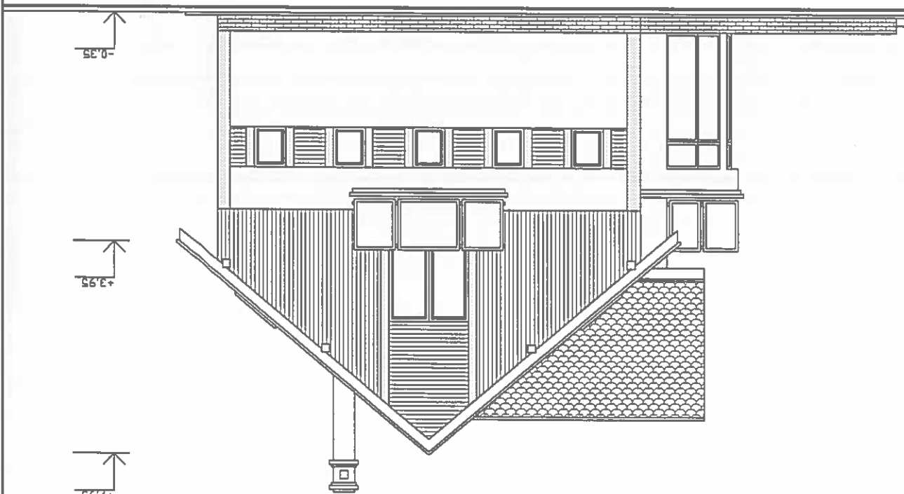
POHLAD SEVEROVÝCHODNÝ
