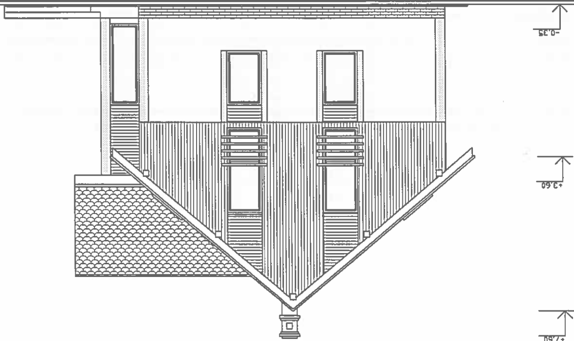
POHLAD SEVEROVÝCHODNÝ
